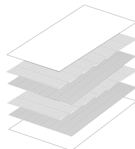
4 pliegues de resina y fibra, consolidados con una película termoplástica para proteger el paquete del compuesto.
